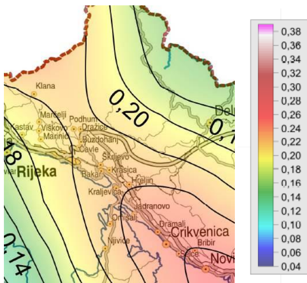
SLIKA 7: IZVOD IZ KARTE POTRESNIH PODRUČJA REPUBLIKA HRVATSKE IZ 2012. GODINE ZA POREDBENO VRŠNO UBRZANJE TLA TIP A S VJEROJATNOSTI PREMAŠAJA 10 % U 50 GODINA ZA POVRATNO ZA POVRATNO RAZDOBLJE TP475 GODINA IZRAŽENO U JEDINICAMA GRAVITACIJSKOG UBRZANJA, (AGR)
